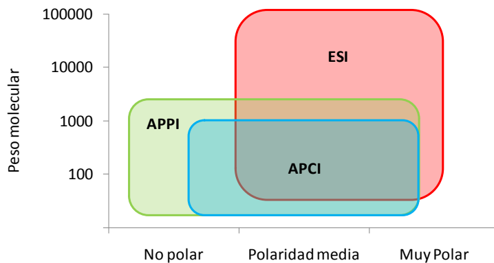
Figura III.12. Rango de aplicación de las fuentes API en función de la polaridad y el peso molecular del analito.
