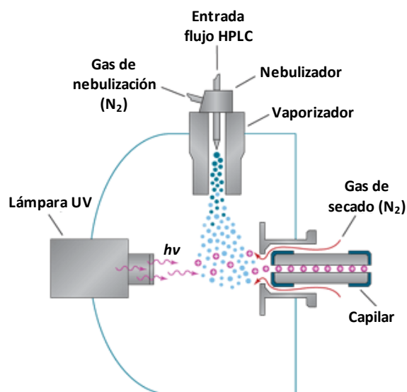
Figura III.16. Esquema de una fuente APPI y proceso de ionización.
